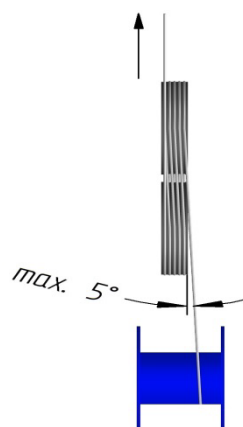
Links geschlagenes Seil
