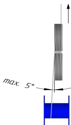
Rechts geschlagenes Seil
